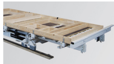
BUILDTEQ A-530
